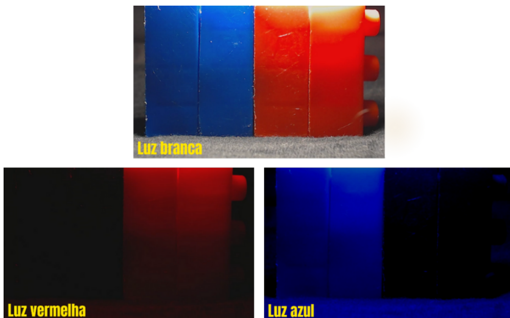
Figura 4.4: Peças de LEGO vermelhas e azuis iluminadas por luzes branca, vermelha e azul.
