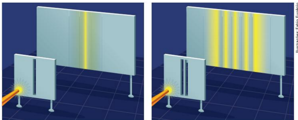
Figura 2.6: Representação do experimento de Young, fora de escala, com fendas simples e duplas (Pietrocola et al. [4]).
