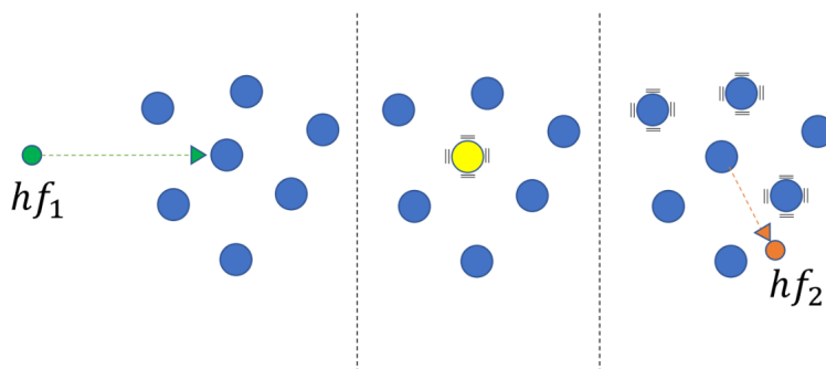
Figura 4.8: Um fóton de energia hf_1 é absorvido por com uma molécula. A molécula perde parte da energia através de interações com moléculas vizinhas e emite o restante na forma de um novo fóton, com energia hf_2 .
