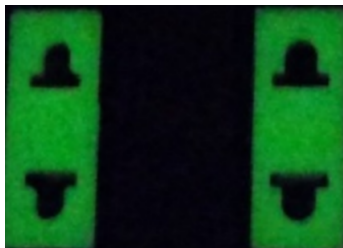
Figura 14: Fosforescência em tomadas antigas.
