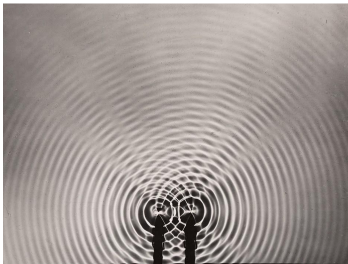
Figura 4.3: Padrão de interferência na cuba de ondas [3].
