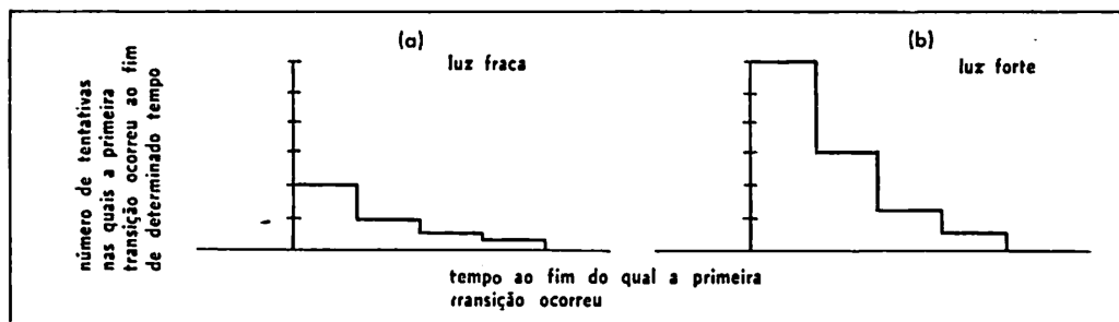
Figura 2.4: Independentemente da intensidade luminosa, os elétrons eram ejetados instantaneamente [3].
