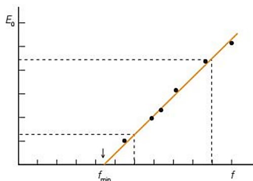
Figura 2.8: Diagrama relacionando a energia máxima do fotoelétron e a frequência da luz [4].
