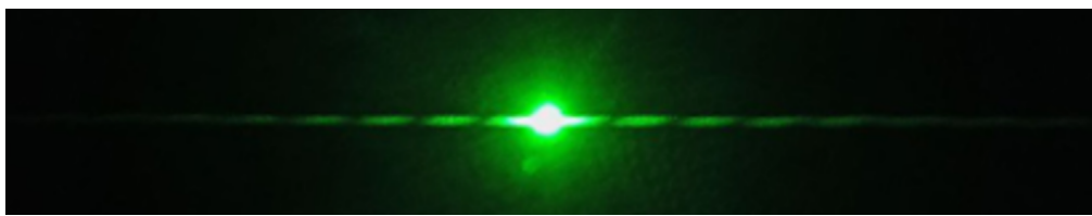
Figura 4: Padrão de claro e escuro formado ao colocarmos o fio de cabelo na frente do feixe de luz.
