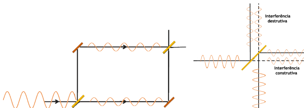
Figura 2.13: À esquerda, os dois caminhos seguidos pelas ondas após separadas pelo primeiro semi-espelho. À direita, a superposição das ondas após o segundo semi-espelho [13].
