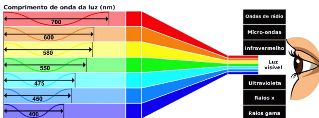
Figura 9: Espectro visível.
