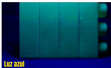
Figura 4.5: Peças de LEGO verdes iluminadas por luz azul.
