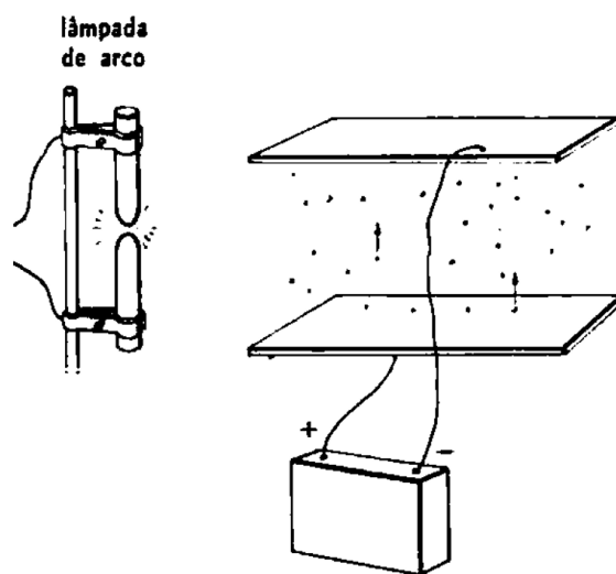
Figura 2.3: As partículas de metal carregadas flutuam entre as placas paralelas sujeitas a uma diferença de potencial. Ao incidir sobre as partículas, a luz arranca-lhes elétrons, fazendo com que as partículas se dirijam para a placa de menor potencial elétrico [3].
