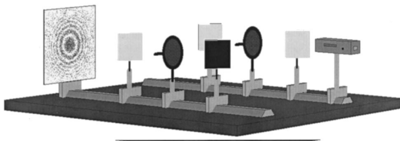
Figura 2.9: Filtros polarizadores paralelos uns aos outros e posicionados nos braços do interferômetro de Mach-Zehnder tornam os caminhos do fóton indistinguíveis, o que produz o padrão de interferência [12].
