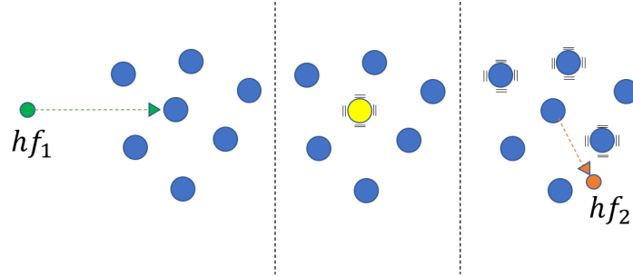
Figura 15: A explicação de Einstein para a fotoluminescência. Um fóton de energia hf_1 é absorvido por uma molécula do corpo fotoluminescente. A molécula perde parte da energia através de interações com moléculas vizinhas e emite o restante na forma de um novo fóton, com energia hf_2 . As pequenas linhas junto às moléculas indicam que estas estão excitadas.
