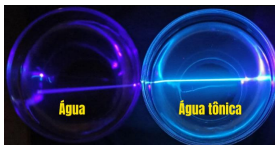
Figura 4.7: Fotoluminescência na água tônica.
