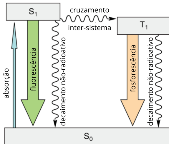
Figura 5.1: Esquema simplificado, traduzido para o português, do diagrama de Perrin-Jablonski mostrando a diferença entre fluorescência e fosforescência. A absorção de um fóton por uma molécula pode levar à formação de um estado excitado pertencente à banda de níveis de energia S_1 , que pode decair ao estado fundamental com a emissão de um fóton por fluorescência ou passar para a banda T_1 , cujos estados têm vida muito mais longa que os de S_1 , e só então decair ao estado fundamental com a emissão de um fóton por fosforescência [7].
