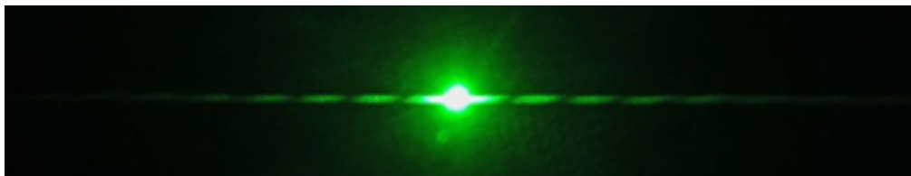
Figura 4.2: Franjas claras e escuras formadas ao iluminar um fio de cabelo com um ponteiro laser .
