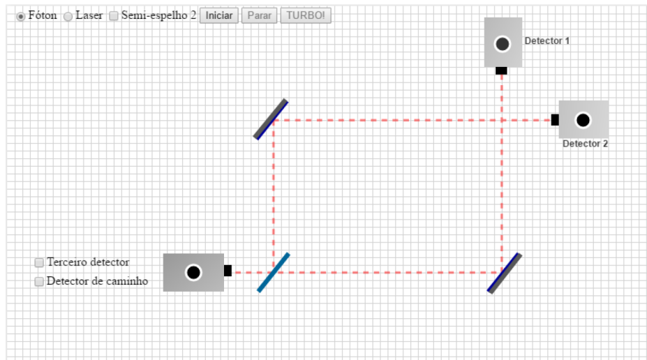
Figura 2.11: Simulação computacional do divisor de luz. A fonte emite luz que atravessa um semi-espelho, podendo ser transmitida ou refletida e, mais a frente, registrada pelos detectores 1 e 2 [13].
