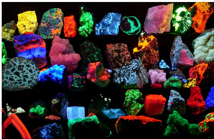
Figura 4.1: Minerais luminescentes iluminados por luz ultravioleta. Foto por Hannes Grobe (Alfred Wegener Institut).
