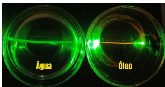
Figura 4.6: Fotoluminescência no óleo de soja.
