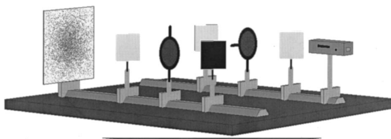
Figura 2.10: Filtros polarizadores perpendiculares uns aos outros e posicionados nos braços do interferômetro de Mach-Zehnder tornam os caminhos do fóton distinguíveis, removendo o padrão de interferência [12].
