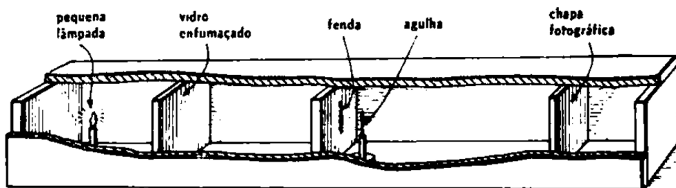
Figura 2.5: Experiência de Taylor para a interferência com luz muito fraca [3].
