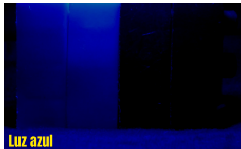
Figura 10: Luz azul iluminando peças de LEGO vermelhas e azuis.
