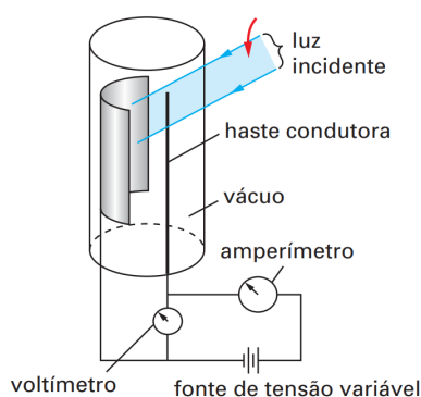
Figura 2.7: Exemplo de esquema para a observação do efeito fotoelétrico [5].
