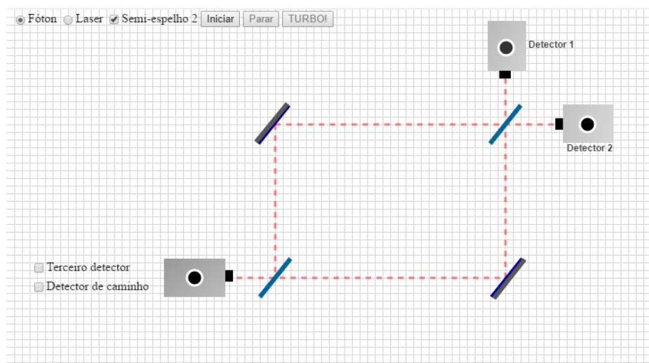
Figura 2.12: Simulação computacional do interferômetro de Mach-Zehnder. A luz em cada braço do interferômetro pode ser transmitida ou refletida pelo semi-espelho posicionado antes dos detectores 1 e 2 [13].
